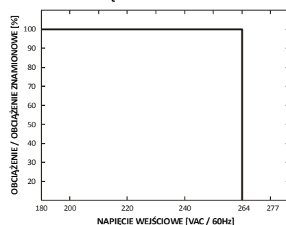
CHARAKTERYSTYKA OBCIĄŻALNOŚCI W ZALEŻNOŚCI OD NAPIĘCIA WEJŚCIOWEGO
