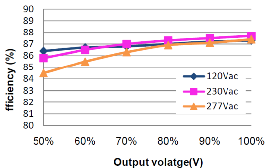
GEHC-070B070 (I = 0.86A)
