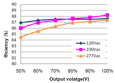
GEHC-060B086 (I = 0.70A)
