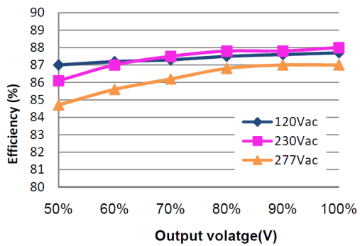
GEHC-060B057 (I = 0.50A)
