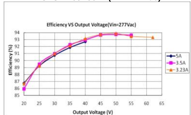
GLUP-200X062Z (Vin=277Vac)
