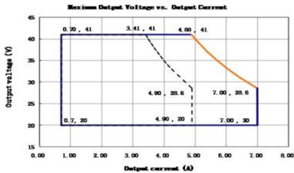
GLUP-200X445Z
