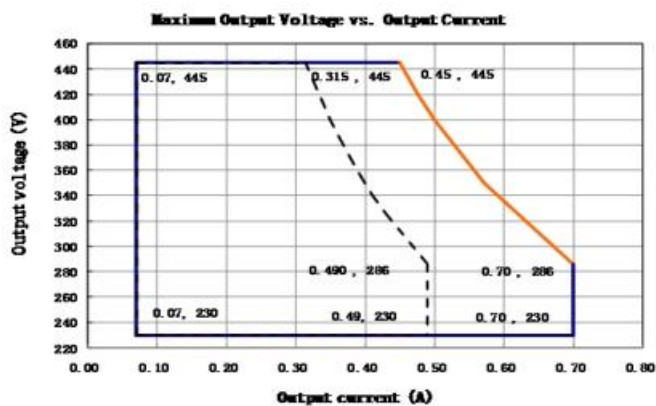
GLUP-200X445Z
