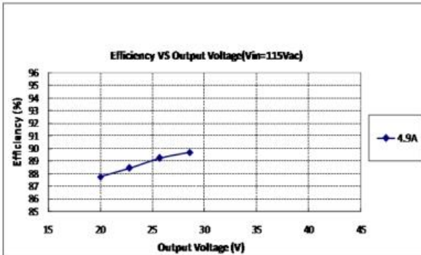
GLUP-200X041Z (Vin=115Vac)
