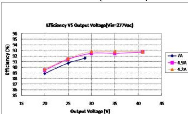
GLUP-200X041Z (Vin=277Vac)
