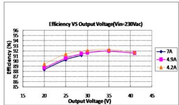
GLUP-200X041Z (Vin=230Vac)
