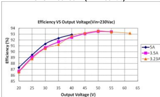
GLUP-200X062Z (Vin=230Vac)
