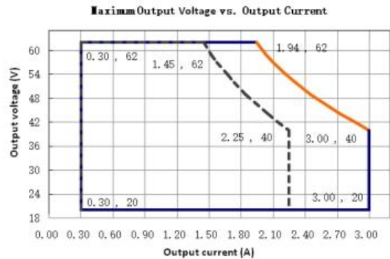
GLUP-120X305Z
