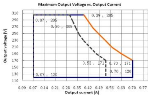
GLUP-120X305Z
