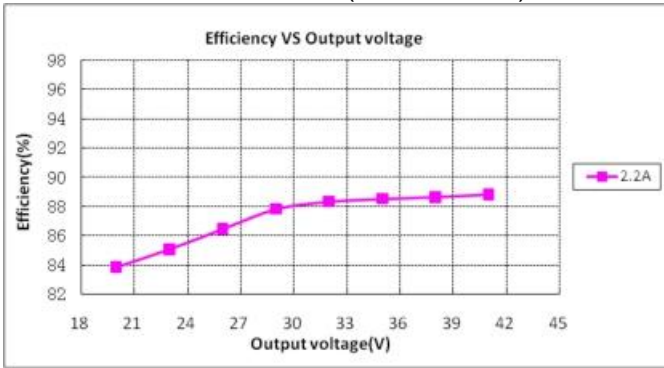
GLUP-120X041Z ( Vin=277Vac )
